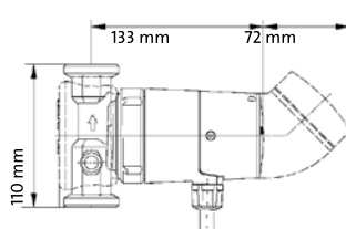
UP 20-14 BX Kompaktný model pre jednoduchú montáž s vonkajším závitom G11/4 a celkovou stavebnou dĺžkou 110 mm
