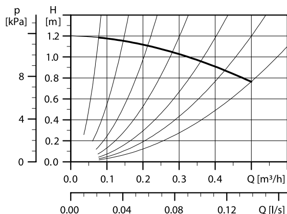
Charakteristická krivka UP 15-14
