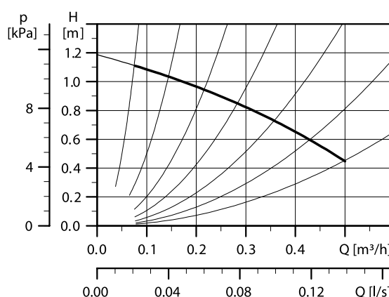
Charakteristická krivka UP 20-14
